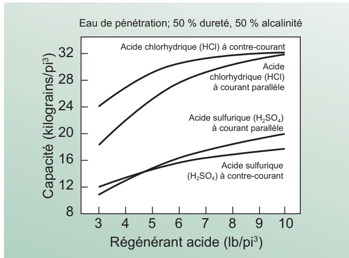
Fig. 4 Capacités opérationnelles typiques de l'Aldex C-800H
