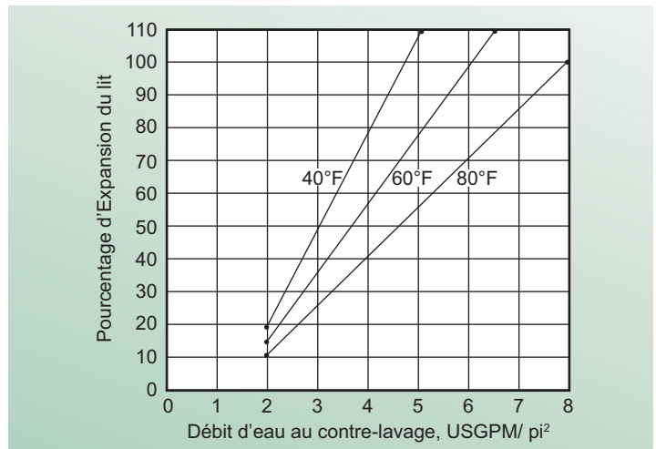
Fig. 2 Expansion du lit vs. Débit de contre-lavage à divers degrés Fahrenheit (F°)
