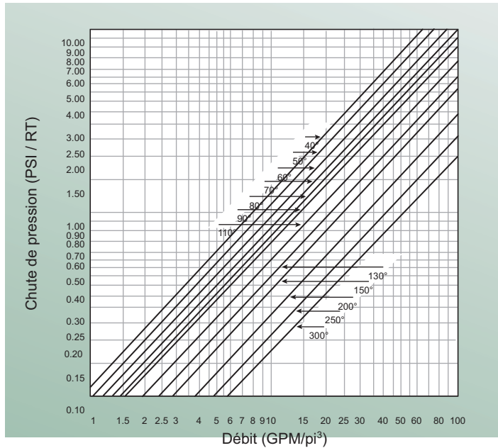
Fig. 1 Chute de pression vs Débit à divers degrés Fahrenheit (F°)
