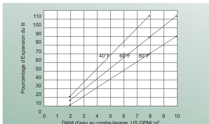
Fig. 2 Expansion du lit vs. débit du contre-lavage pour diverses températures d'eau
